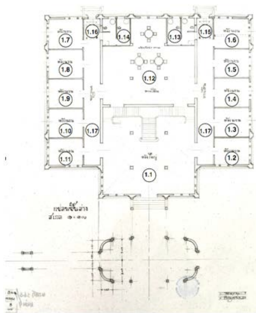
ภาพที่ 12 แล่นชั้นที่ 1 พระที่นั่งอุดมวนาภรณ์ (อยู่ด้านขวา ของพระที่นั่งไวกูณฐเทพยสถาน) ที่มา : หอจดหมายเหตุแห่งชาติ 1.6.5/2
