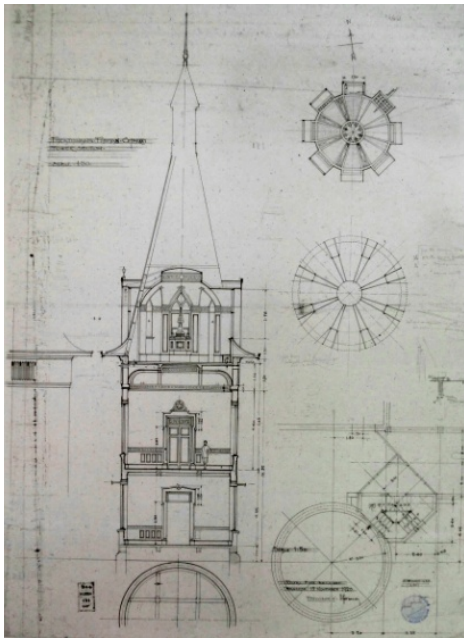
ภาพที่ 7 แบบขยาย แปลน รูปตัด หอสูง พระที่นั่งพิมานจักรี ที่มา : หอจดหมายเหตุแห่งชาติ ผ กสก 1.6.2/3
