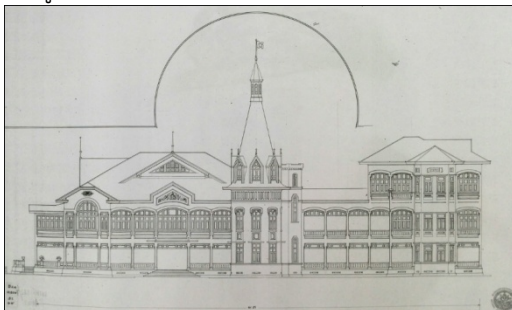
ภาพที่ 4 แบบรูปด้านทิศใต้พระที่นั่งพิมานจักรี (ด้านซ้าย) และ พระที่นั่งไวกูณฐเทพยสถาน (ด้านขวา) ที่มา : หอจดหมายเหตุแห่งชาติ ผ กสก 1.6.5/5
