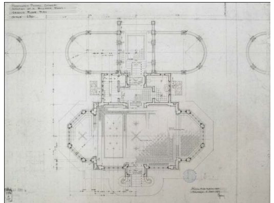
ภาพที่ 13 แล่นพื้นชั้นที่ 1 ห้องบิลเลียด (หรือห้องรับรอง) ชั้นบนเป็นดาดฟ้า ที่มา : หอจดหมายเหตุแห่งชาติ ผ. กสก 1.6.5/2
