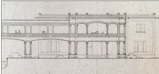
ภาพที่ 11 แบบรูปด้านทิศใต้ พระที่นั่งอุดมวนาภรณ์ ที่มา : หอจดหมายเหตุแห่งชาติ 1.6.5/2
