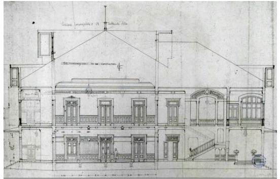
ภาพที่ 5 รูปตัดแนวทิศเหนือ-ทิศใต้ พระที่นั่งพิมานจักรี ที่มา : หอจดหมายเหตุแห่งชาติ ผ กสก 1.6.2/1 ในแบบระบุปี ค.ศ. 1920 (หรือ พ.ศ. 2463)
