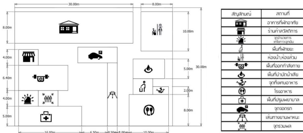
ภาพ 1 แผนผังที่ตั้งของอาคารในพื้นที่จัดสวัสดิการอาคารที่พักอาศัยสำหรับแรงงานก่อสร้าง ที่มา: ผู้วิจัย
