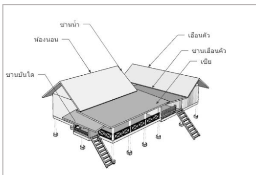
ภาพ 12 จำลองการปิดล้อมเชียนดั้งเดิม (ที่มา: ผู้วิจัย, 2563)
