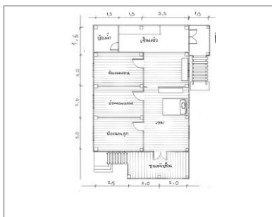
ภาพ 16 ผังพื้นเอื้อนรูปแบบใหม่หลังที่ 117 (ที่มา: ผู้วิจัย, 2563)
