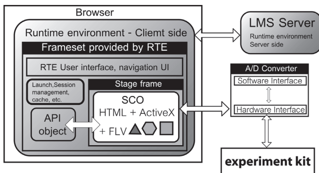
ภาพที่ 4 การทำงานของระบบรับสัญญาณจากชุดทดลองเพื่อแสดงผลและส่งข้อมูลไปยังระบบจัดการการเรียนรู้
