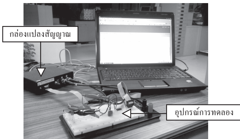
ภาพที่ 2 ระบบการเรียนการสอนปฏิบัติการผ่านเครือข่ายระบบจัดการการเรียนรู้ มาตรฐานสกอর্মฝั่งผู้เรียน
