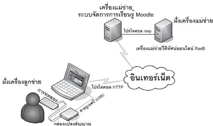
ภาพที่ 1 สถาปัตยกรรมระบบการเรียนการสอนปฏิบัติการผ่านเครือข่ายระบบจัดการ การเรียนรู้มาตรฐานสกอ
