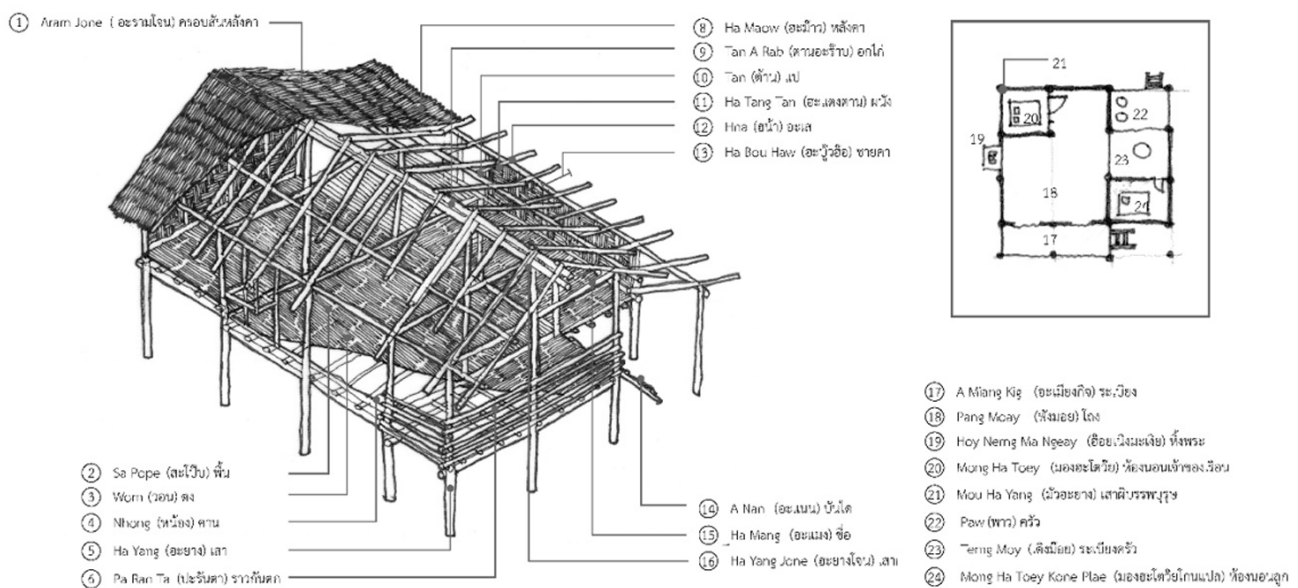
ภาพที่ 2 ภาพไอโซเมตริกและผังพื้นแสดงลักษณะเรือนในสมัยเริ่มตั้งถิ่นฐานของชาวมอญชุมชนดงสัก
