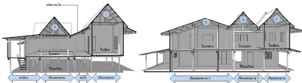
ภาพที่ 9 ซ้าย: รูปตัดเรือนแบบ 2 จั่วร่วมพื้น ขวา: รูปตัดเรือนแบบ 3 จั่วร่วมพื้น
