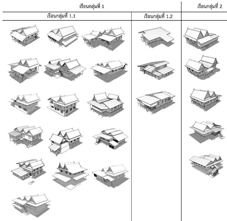
ภาพที่ 3 เรือนกรณีศึกษา 24 หลัง ที่มีความเด่นชัดของเป็นกลุ่มเรือนไทย-ยวนคูบัว
