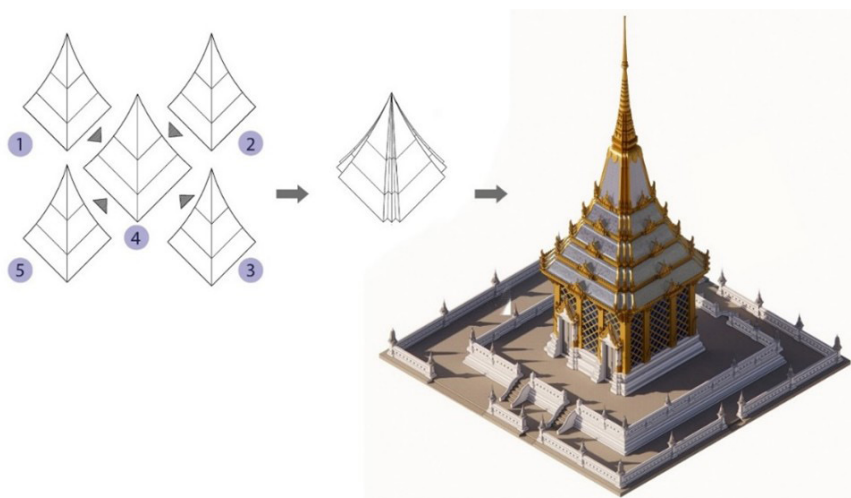
ภาพที่ 13 ภาพสามมิติแสดงแนวคิดและรูปทรงหลังคามณฑปพระพุทธรูป (แบบที่ 2) (ที่มา : Tawan Weerakoon)
