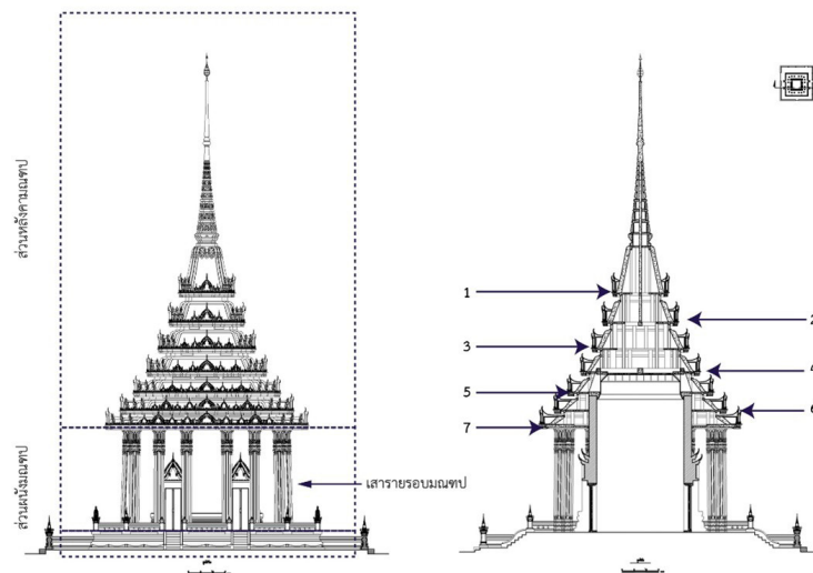
ภาพที่ 1 แบบรูปด้าน มณฑปพระพุทธบาทสระบุรี (ซ้าย) และรูปตัดแสดงชั้นเชิงกลอน 1-7 มณฑปพระพุทธบาทสระบุรี (ขวา) (ที่มา : Tawan Weerakoon)
