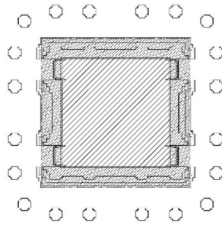
ภาพที่ 4 ลายเส้นเปรียบเทียบระหว่างพื้นที่ภายในและภายนอกมณฑปพระพุทธรูปจากการประมาณการของ Jacobus van den Heuvel (เส้นแรเงาแสดงพื้นที่ภายใน 7.31 x 7.31 ตารางเมตร เส้นแรเงาที่แสดงพื้นที่ภายนอก 9.9 x 9.9 ตารางเมตร) กับพื้นที่ภายในมณฑปพระพุทธรูปปัจจุบัน (ที่มา : Tawan Weerakoon)
